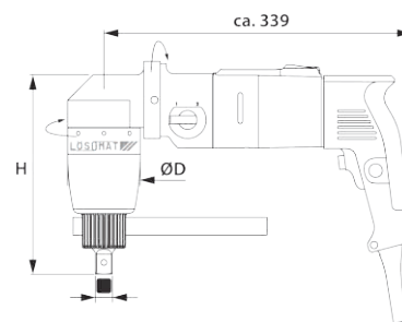
LEW-S elektrisch
