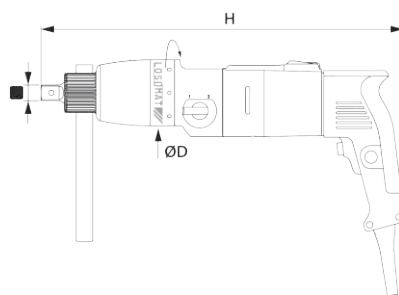
LDE-S elektrisch
